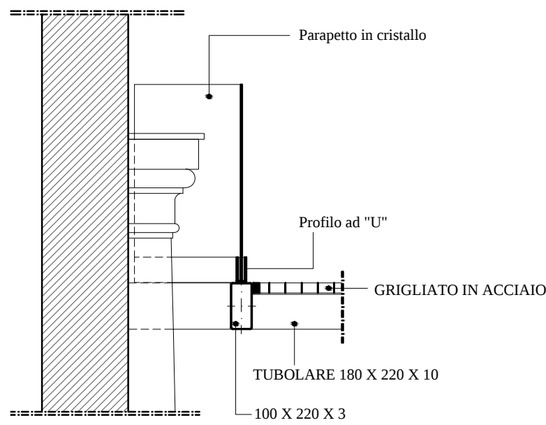
Sezione C-C
